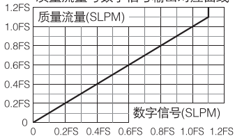
质量流量与数字信号输出对应曲线
