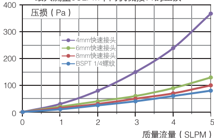
最大流量5SLPM不同机械接口的压损
