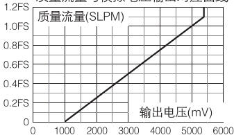
质量流量与模拟电压输出对应曲线
