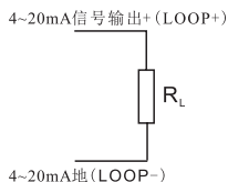
(图6-2) 4~20mA信号输出外部接线图
