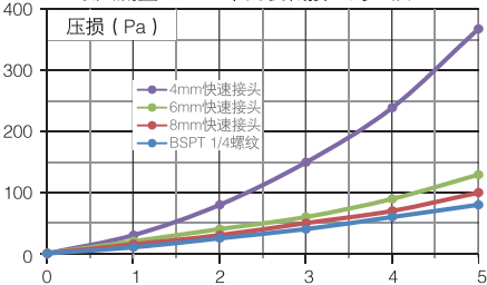
最大流量5SLPM不同机械接口的压损
