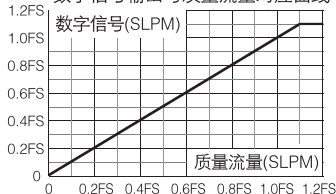
数字信号输出与质量流量对应曲线
