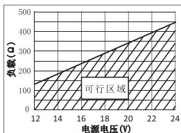
(图6-6) 负载与电源电压关系图
