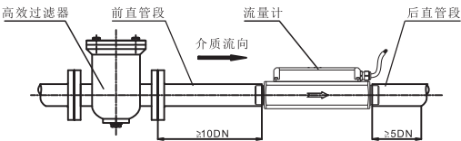
(图5-3) 流量计管道安装示意图
