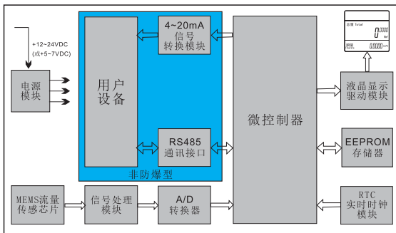
(图3-2) 流量计原理框图
