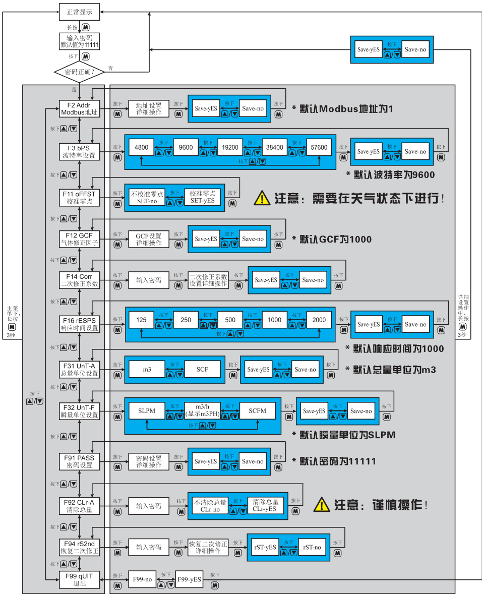
(图6-10) 按键操作流程图
