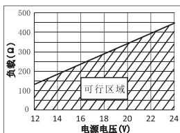
(图6-6) 负载与电源电压关系图
