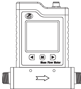
（图6-7）用户界面
