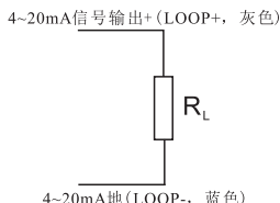
(图6-5) 4~20mA信号输出外部接线图
