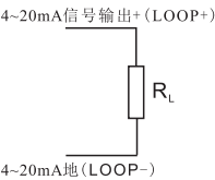
（图6-2）4~20mA信号输出外部接线图
