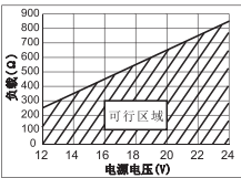
（图6-3）负载与电源电压关系图
