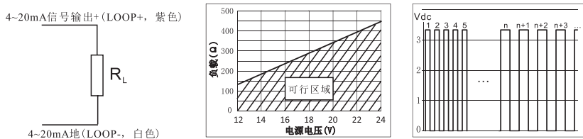
(图6-6) 4~20mA信号输出外部接线图 (图6-7) 负载与电源电压关系图 (图6-8) 脉冲输出波形图
