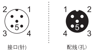
接口(针)
