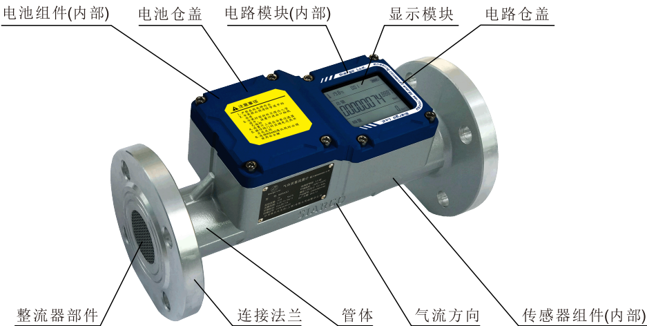
产品结构图
