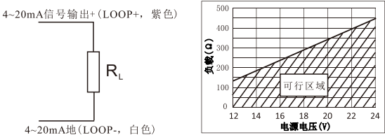
(图6-6) 4~20mA信号输出外部接线图
