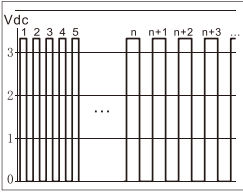
(图6-8) 脉冲输出波形图
