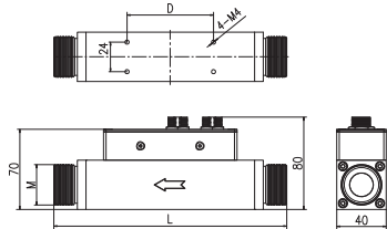
流量计主体
