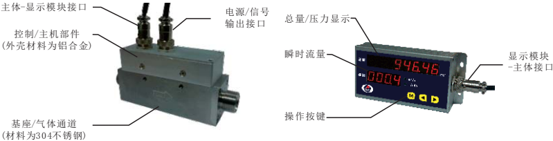
(图3-1) 流量计主体结构图
